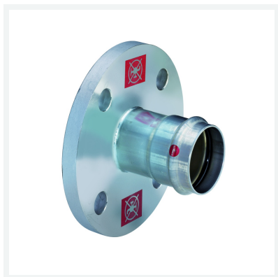
Prestabo karimás átmeneti idom SC-Contur-ral (biztonsági kontúr) modellszám 1159 cikkszám 643 560
